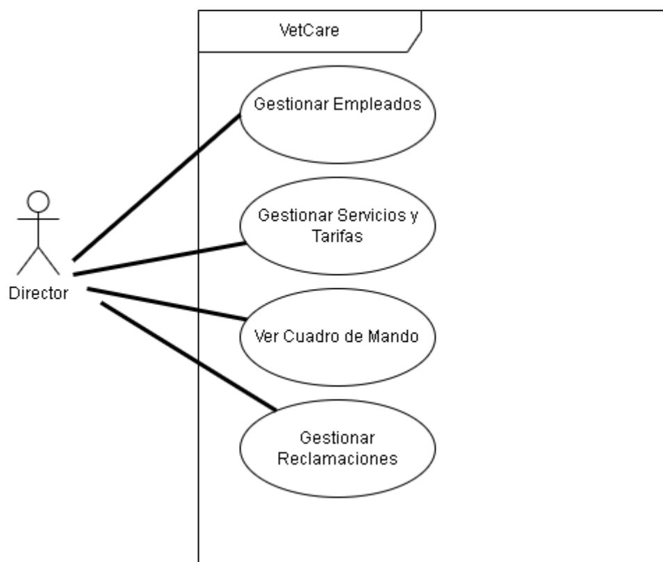
Diagrama de casos de uso del rol Director
