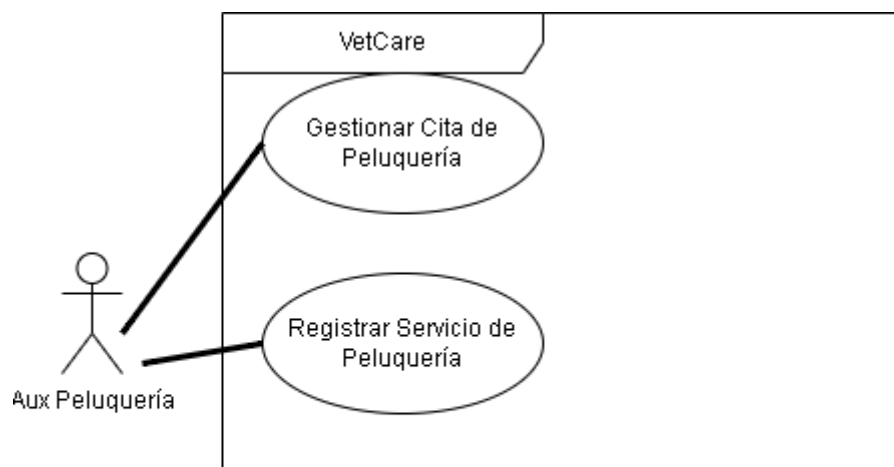
Diagrama de casos de uso del Rol Aux.Peluquería
