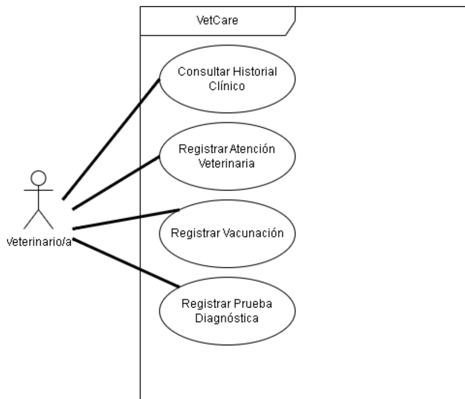
Diagrama de casos de uso del Rol Veterinario
